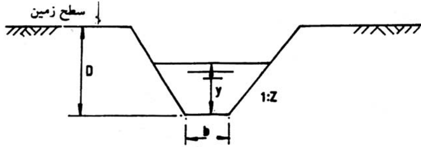
شکل ۶-۱. مقطع عرضی تیپ یک نهر زهکشی
